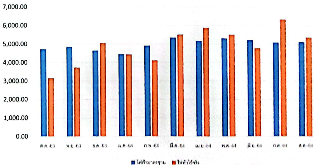
แผนภูมิที่ ๑ สถิติการใช้พลังงานไฟฟ้า เปรียบเทียบกับค่ามาตรฐานการใช้พลังงาน
